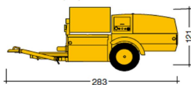
DIMENSIONI (cm)
